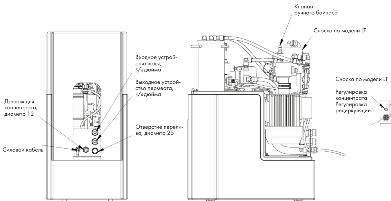
Рисунок 1. Фитинги для подключения воды и клапаны на BWT bestaqua 60
